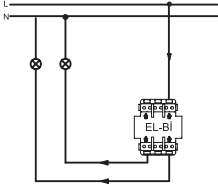
Выключатель кнопочный 2-кл XXX-XXXXXX-257
