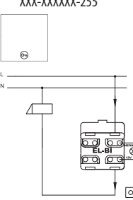
Кнопка дверной автоматики с подsv. XXX-XXXXXX-255
