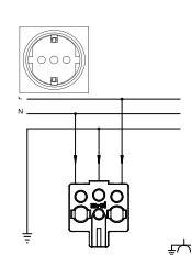
Розетка с защитной шторкой с/з XXX-XXXXXX-243
