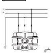
Регулятор вентилятора XXX-XXXXXX-277 (110 V) (200W) XXX-XXXXXX-278 (220 V) (200W)
