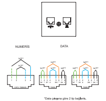
Розетка компьютерная + телефон XXX-XXXXXX-249
