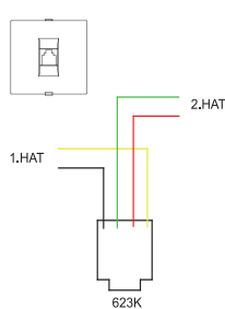
Розетка телефонная XXX-XXXXXX-221
