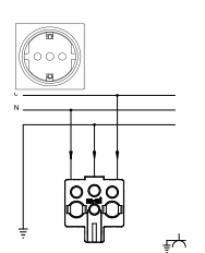
Розетка с защитной крышкой с/з XXX-XXXXXX-218
