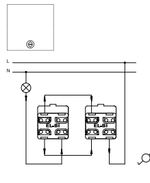
Выключатель 1-кл проходной XXX-XXXXXX-209
