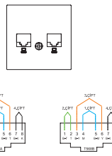
Розетка компьютерная двойная XXX-XXXXXX-248
