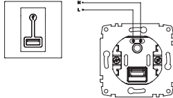
Розетка USB XXX-XXXXXX-142 (Zena)
