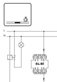
Выключатель кнопочный с подств. Led XXX-XXXXXX-206
