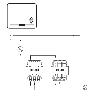
Выключатель 1-кл проходной с подств. Led XXX-XXXXXX-210
