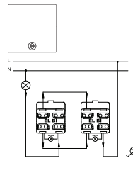
Выключатель 1-кл проходной с подsv. Led XXX-XXXXXX-210
