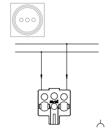
Розетка компьютерная + телефон XXX-XXXXXX-249
