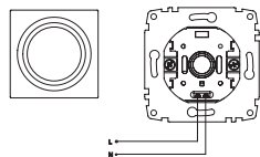
Подсветка ориентационная (Led) с выключателем XXX-XXXXXX-185 (Zena)
