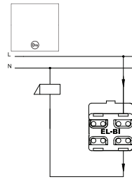
Выключатель 1-кл проходной с подsv. Led XXX-XXXXXX-210
