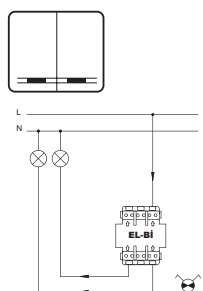
Выключатель 2-кл с подств. Led XXX-XXXXXX-203
