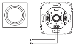
Подсветка ориентационная (Led) XXX-XXXXXX-184 (Zena)
