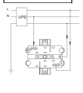
Подсветка ориентационная (Led) XXX-XXXXXX-184 (Zena)
