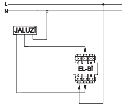
Выключатель для жалюзи 3 позиции XXX-XXXXXX-297
