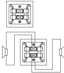
Розетка Hi-Fi двойная XXX-XXXXXX-241
