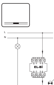
Выключатель 1-кл с подств. Led XXX-XXXXXX-201
