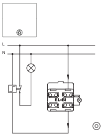
Выключатель кнопочный с подsv. Led XXX-XXXXXX-206
