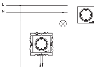
Диммер 600W XXX-XXXXXX-113
